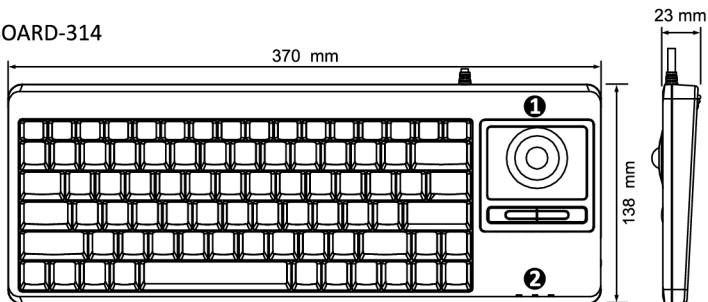
PERIBOARD-315
