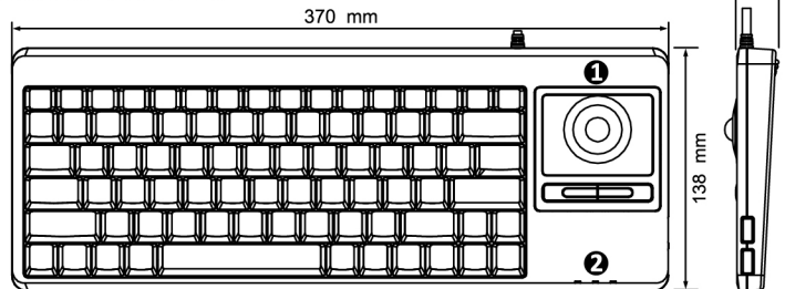
PERIBOARD-315 + 2Hubs
