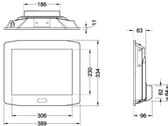
MES 1215PC 389*96*334(mm) - Built-in AC adapter
