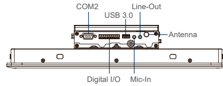
Right I/O
