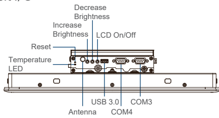
Left I/O
